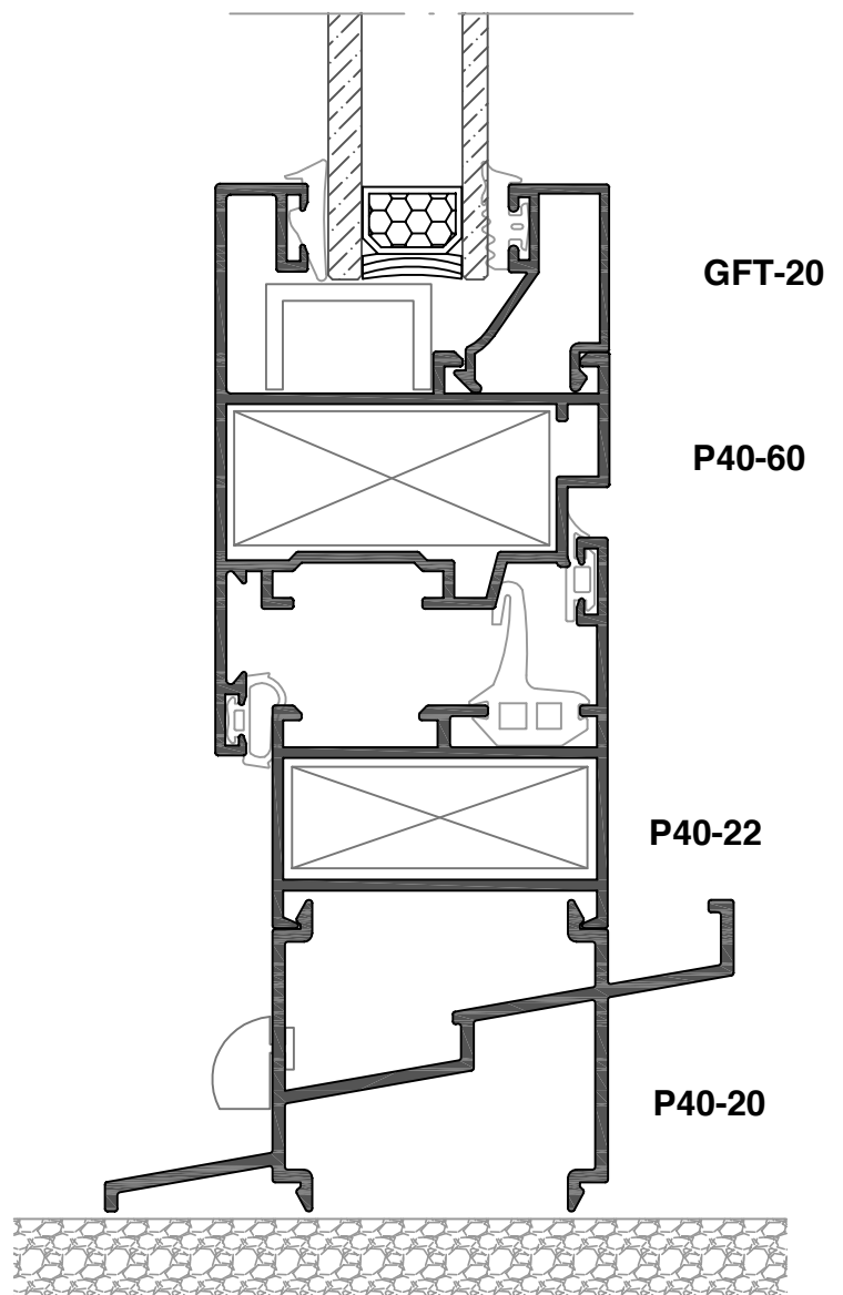
Corte 11
