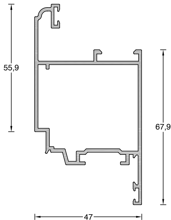
P40-60 Hoja ventana apertura exterior
