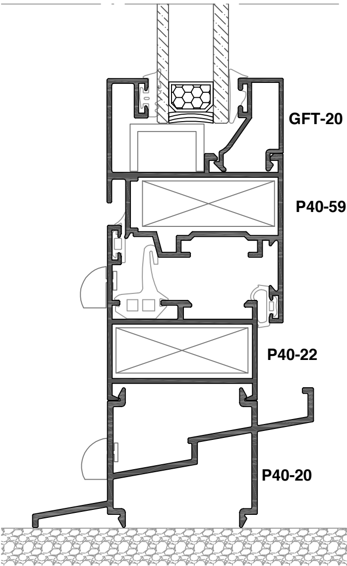
Corte 3
