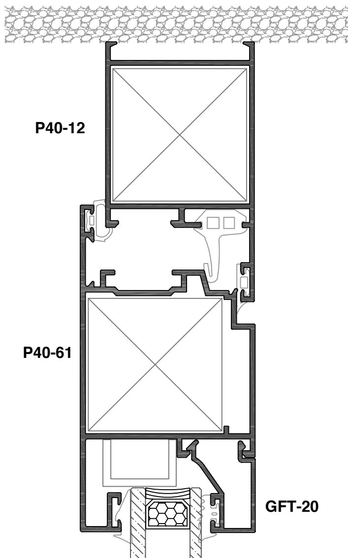
Corte 16
