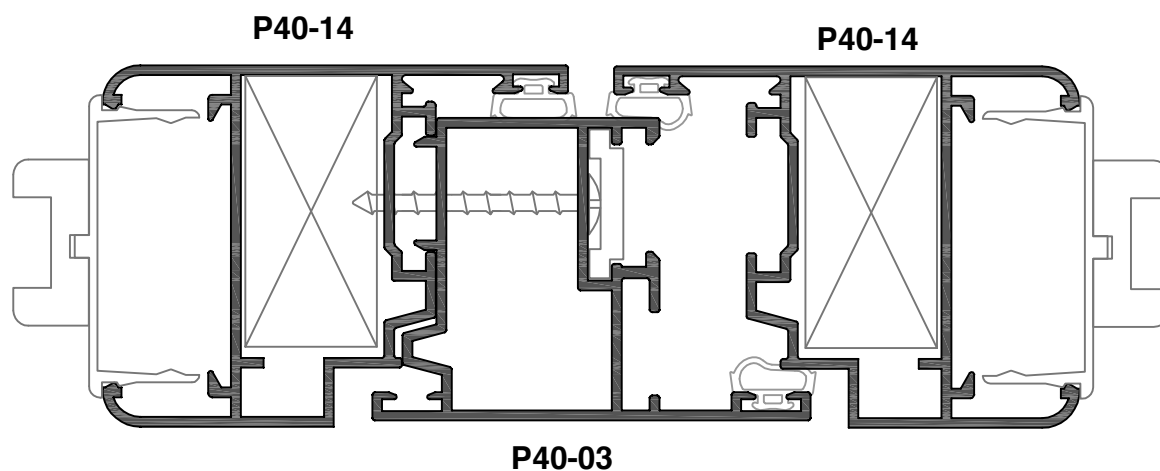
Corte 26
