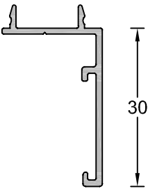
GALI-1117V Solape 45 mm para marco
