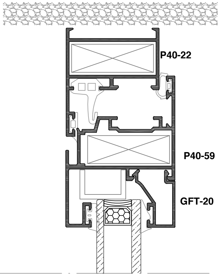
Corte 1
