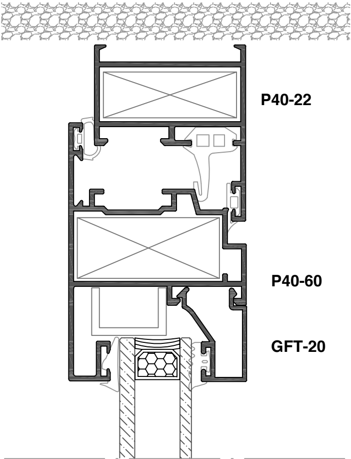
Corte 5
