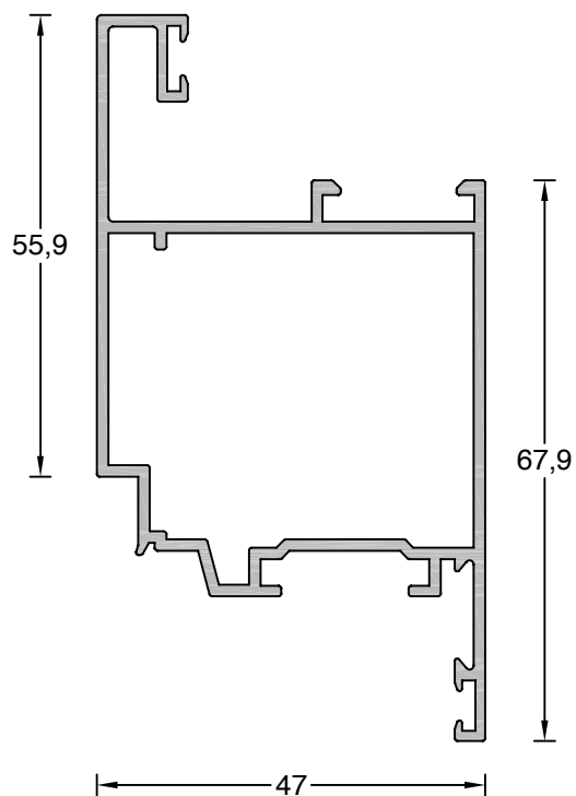
P40-05R Hoja ventana apertura exterior
