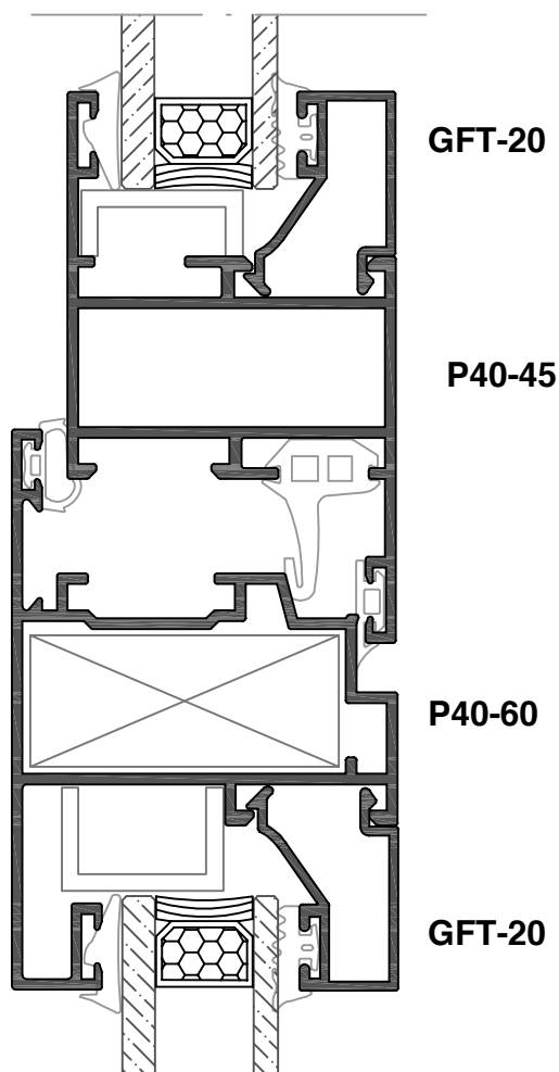
Corte 9
