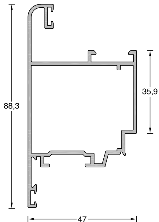
P40-06 Hoja puerta apertura exterior
