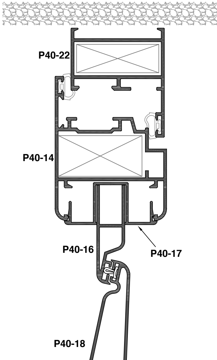
Corte 20
