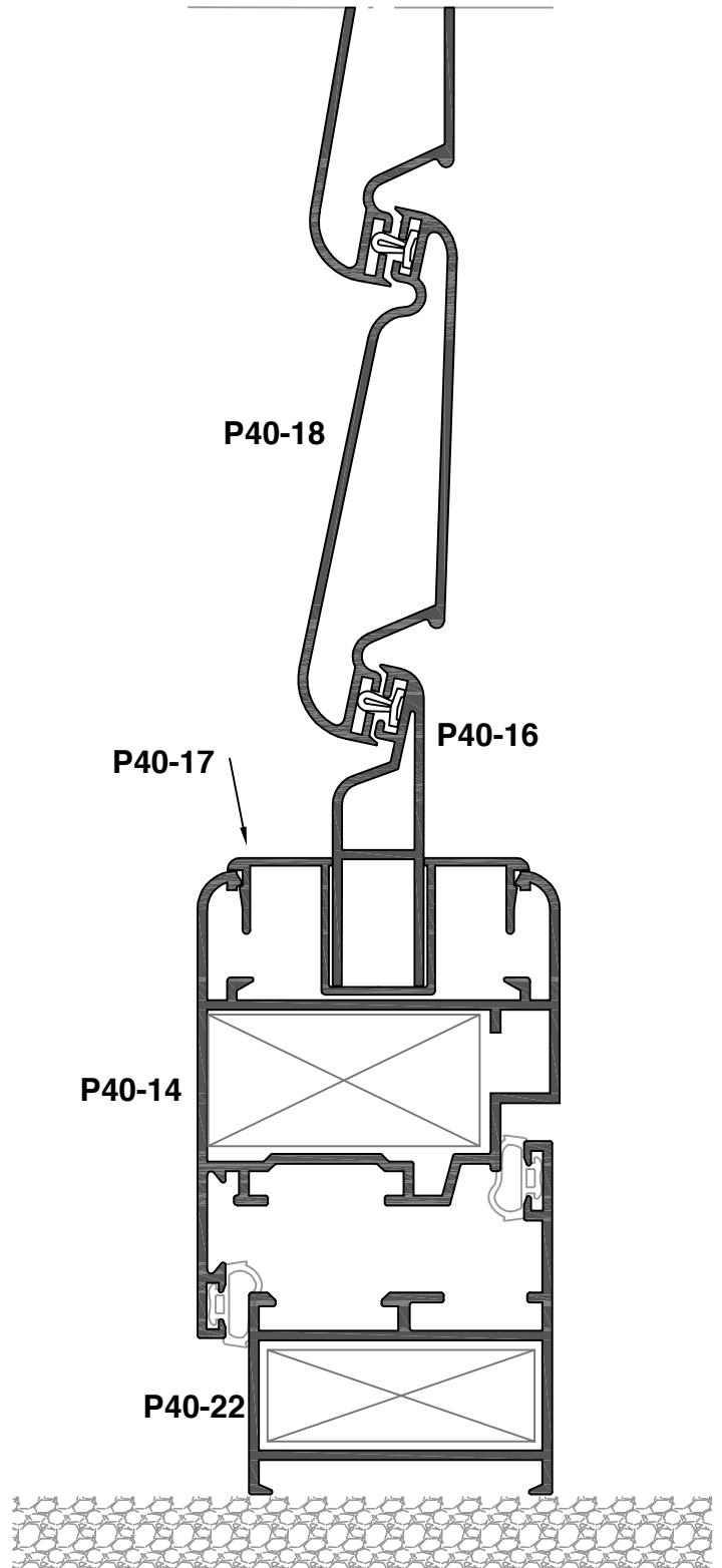
Corte 22
