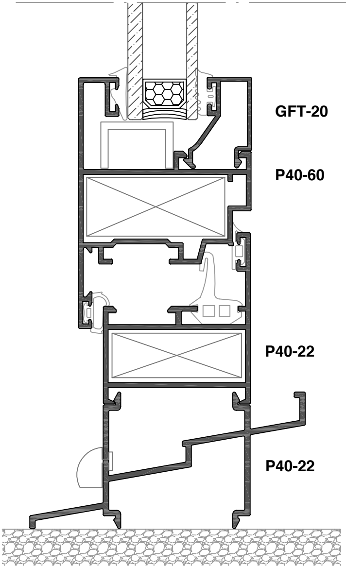
Corte 7
