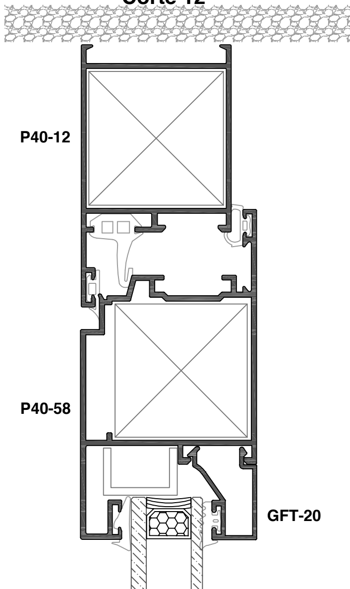
Corte 12
