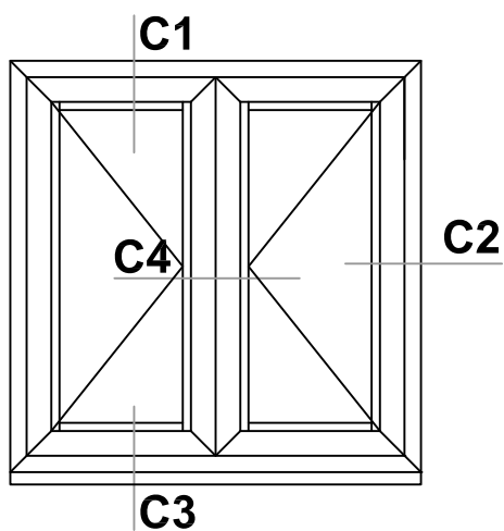
Ventana 2 hojas apertura interior
