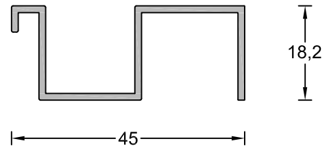
S-01N Guía persiana
